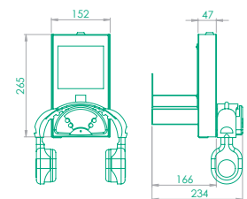
B Borne d'écoute Monolux (1 CD) PE1CD
