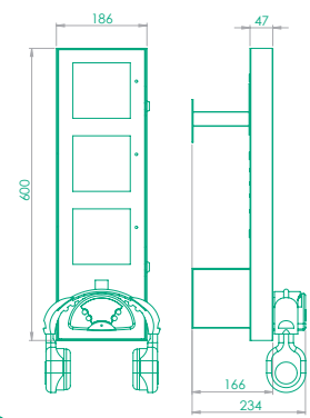
A Borne d'écoute Multi (3 CDs) PE3CD
