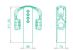
D Borne d'écoute à la demande BEA
