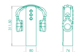
C Borne d'écoute MP3 PEMP3
